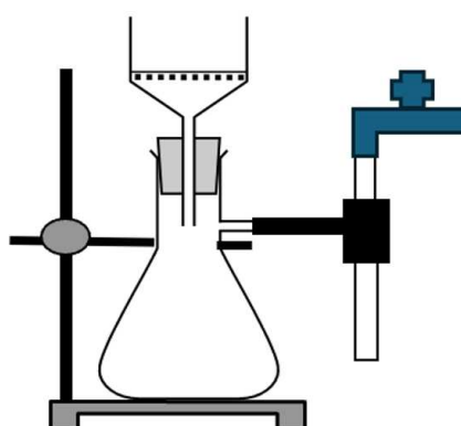
Montage B
