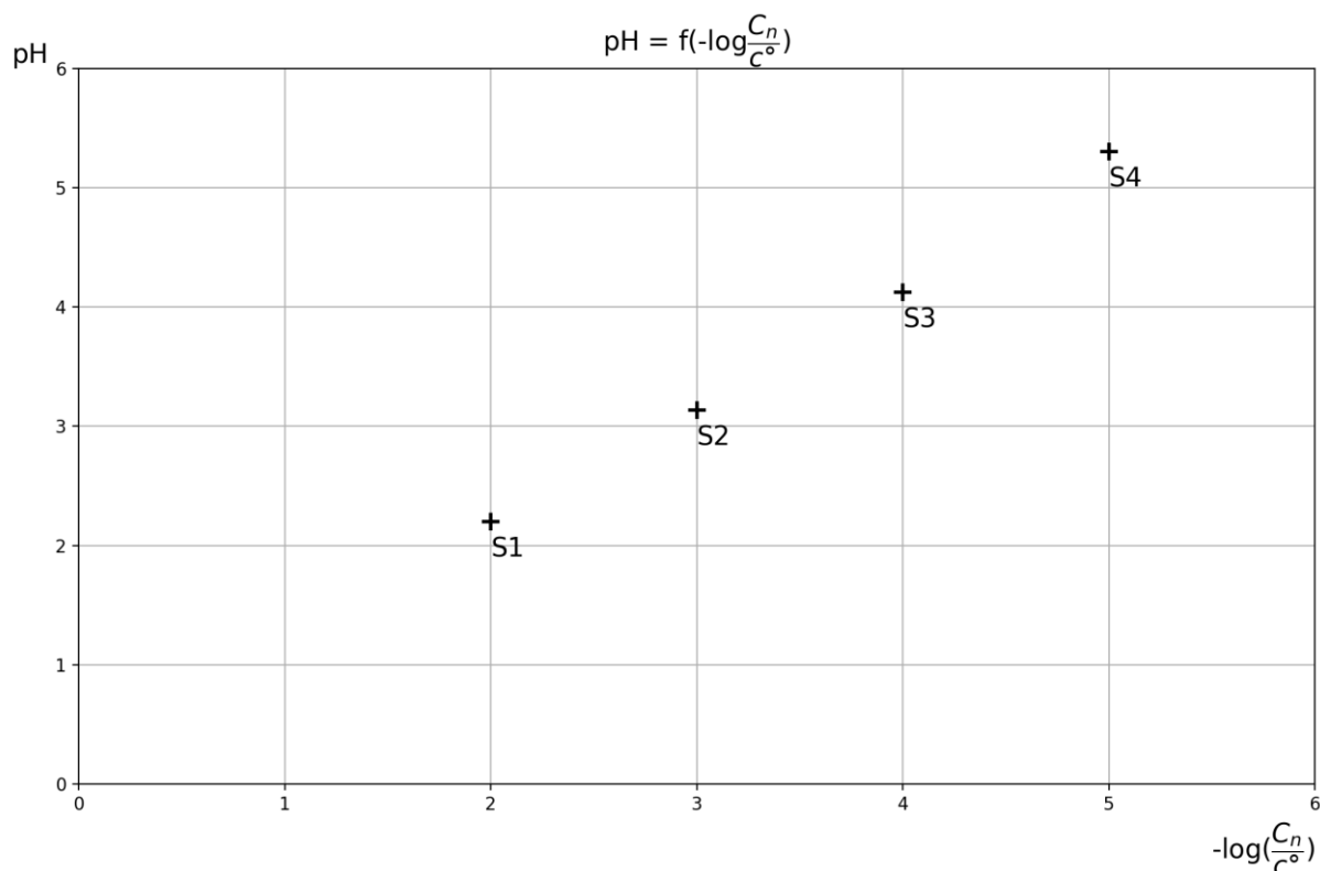
Figure 2. Évolution de la valeur du pH en fonction de -\log(\frac{C_n}{C^o})
