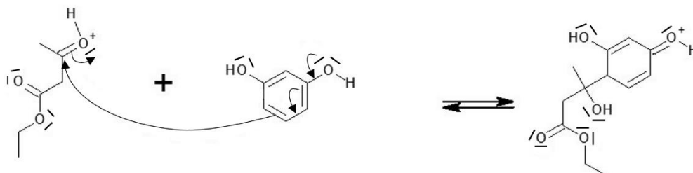
Figure 4. Les deux premières étapes du mécanisme de la synthèse
