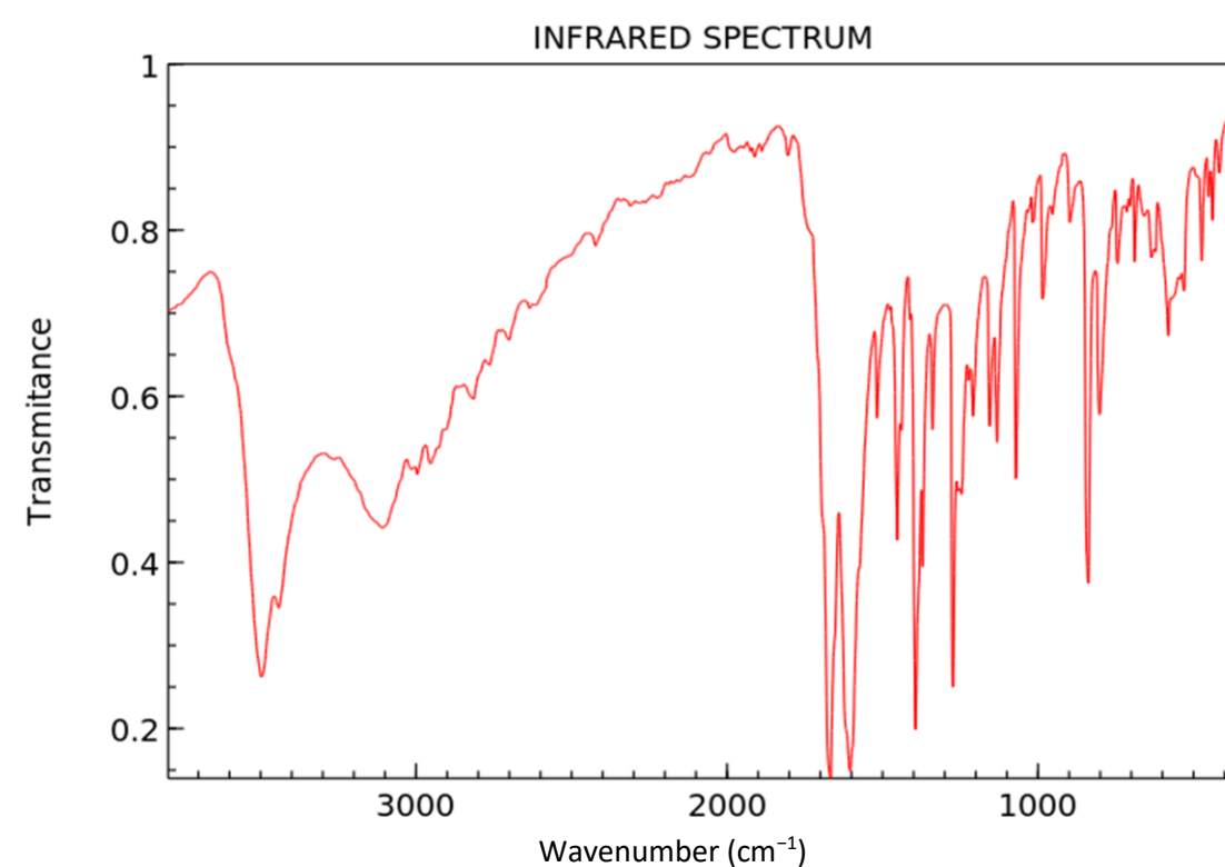
Figure 3. Spectre infrarouge du produit obtenu
