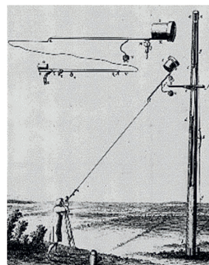
La lunette à fil tendu Dessin de C. Huygens
