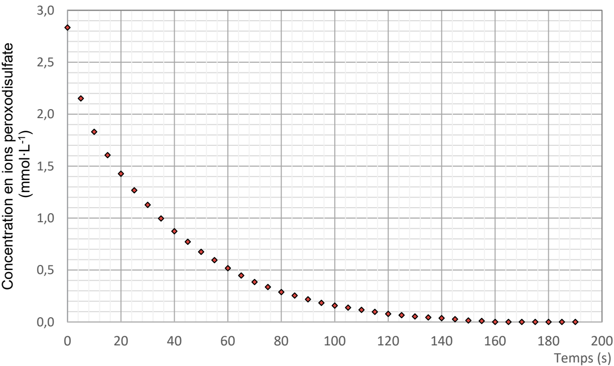
Figure 3. Évolution de la concentration en ions peroxodisulfate en fonction du temps
