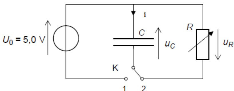
Figure 3 : Schéma du circuit électrique
