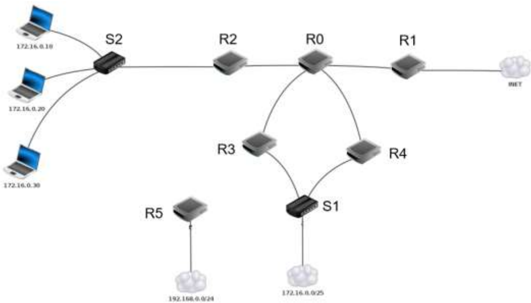
Figure 2. Architecture Réseau
