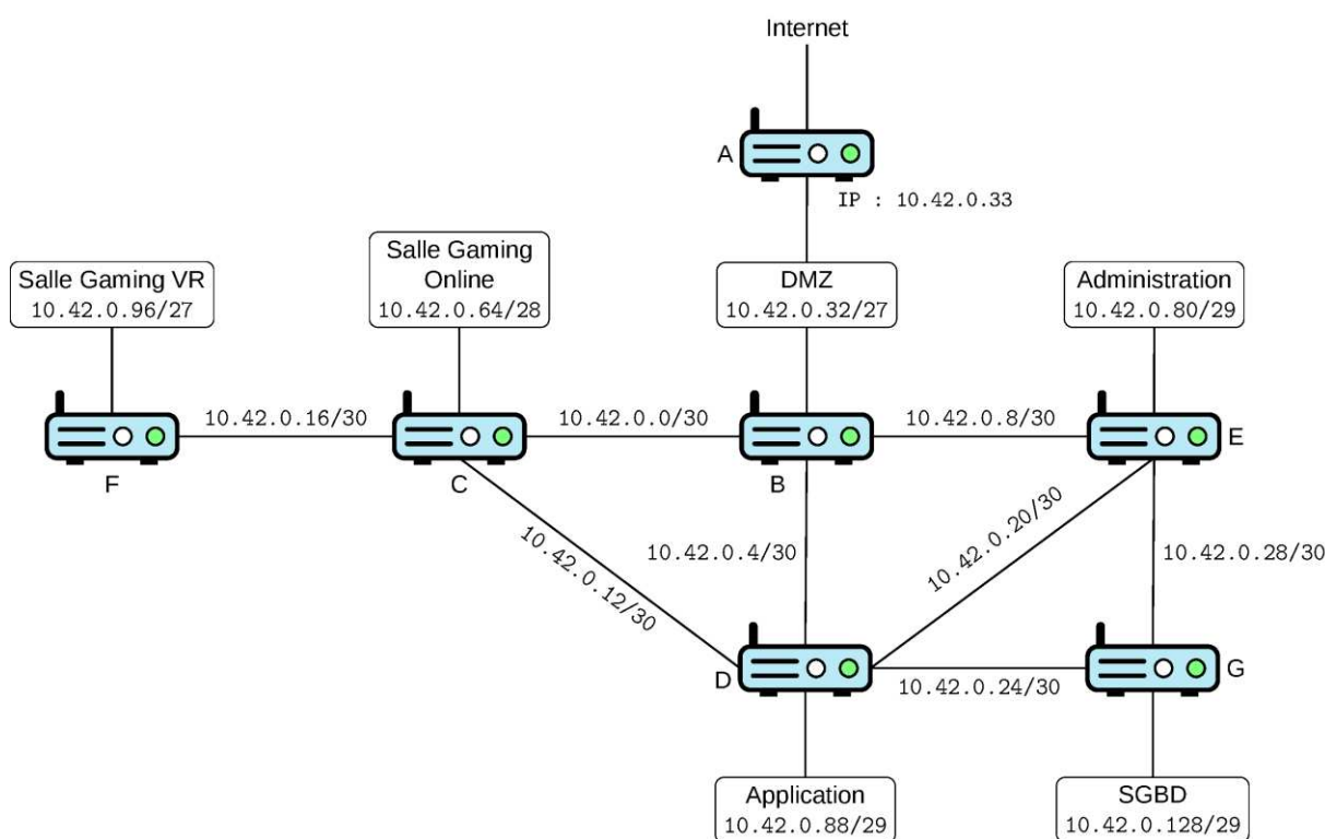
Figure 1. Réseau de l'entreprise Gamerzz
